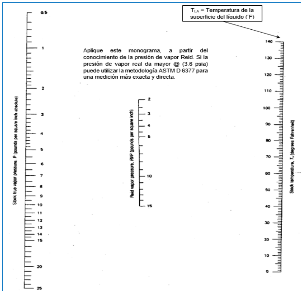
Figura. 7.1-13a Nomograma para cálculo de la presión de vapor real.
